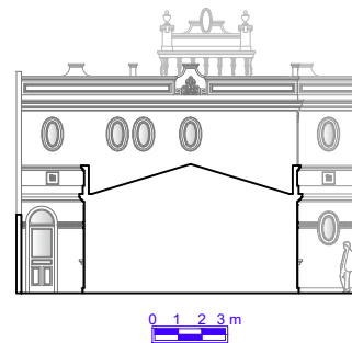
Elevação 03
